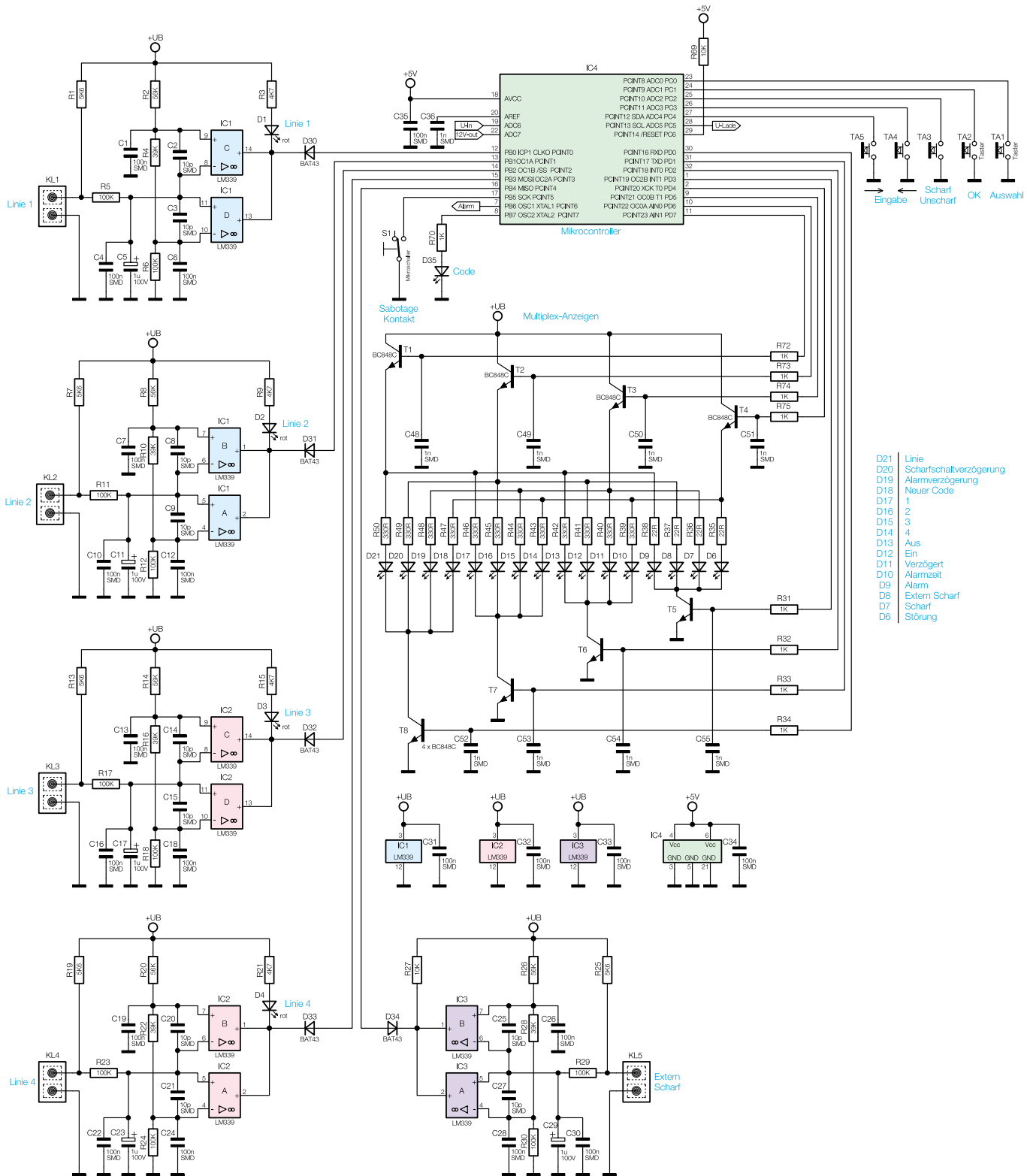
Bild 6: Hauptschaltbild der Alarmzentrale AZ-2
