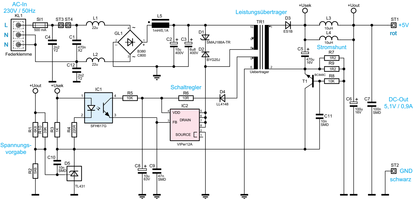
Bild 1: Schaltplan des Netzteils für die Unterputz-Montage
