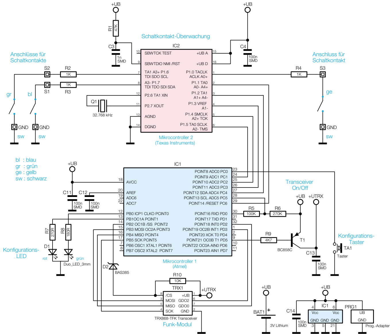
Bild 2: Schaltung des HM-SCI-3-FM
