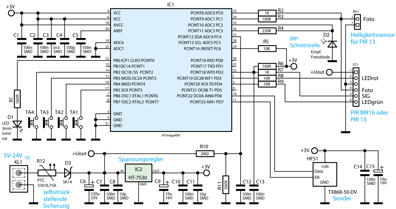
Bild 6: Die Schaltung des FS20 SPIR-LUX
