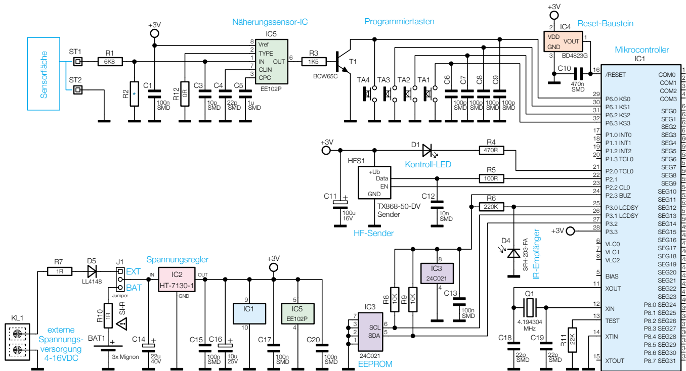
Bild 2: Das Hauptschaltbild des FS20 TC1
