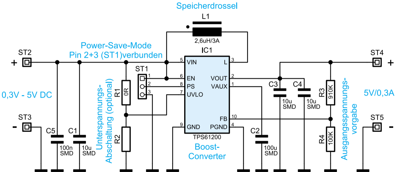
Bild 7: Schaltung des SBC 300
