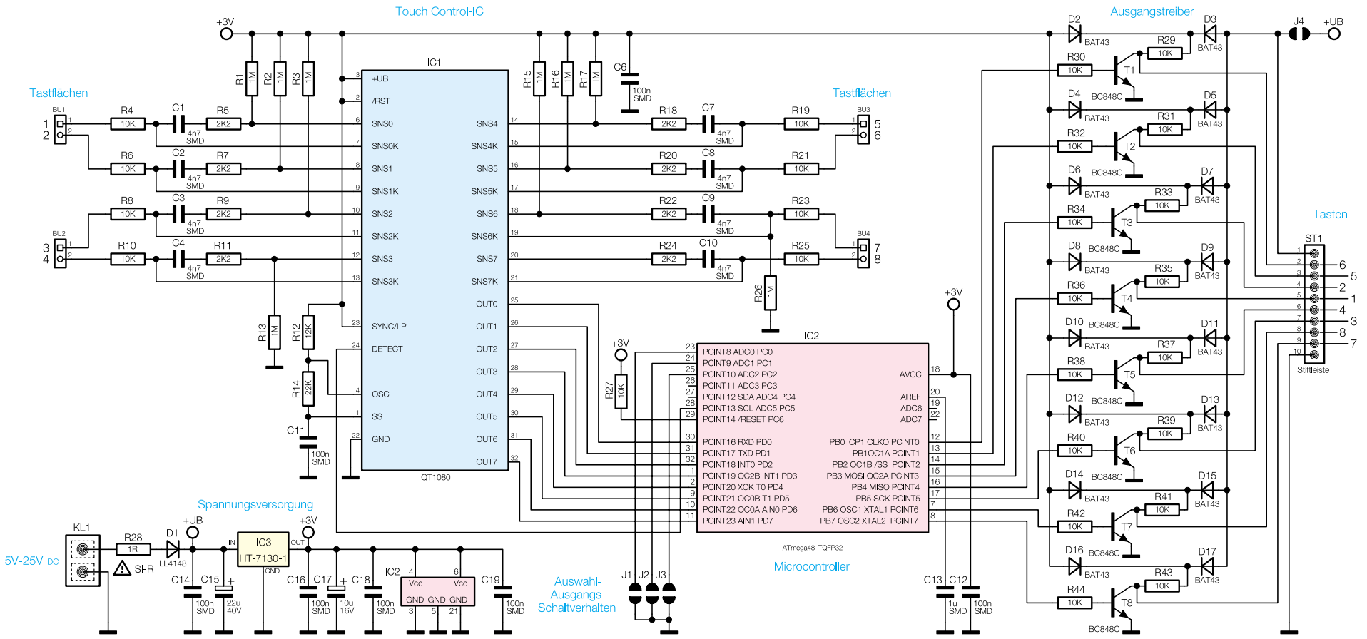
Bild 3: Schaltbild des Touch-Control-Moduls TC8
