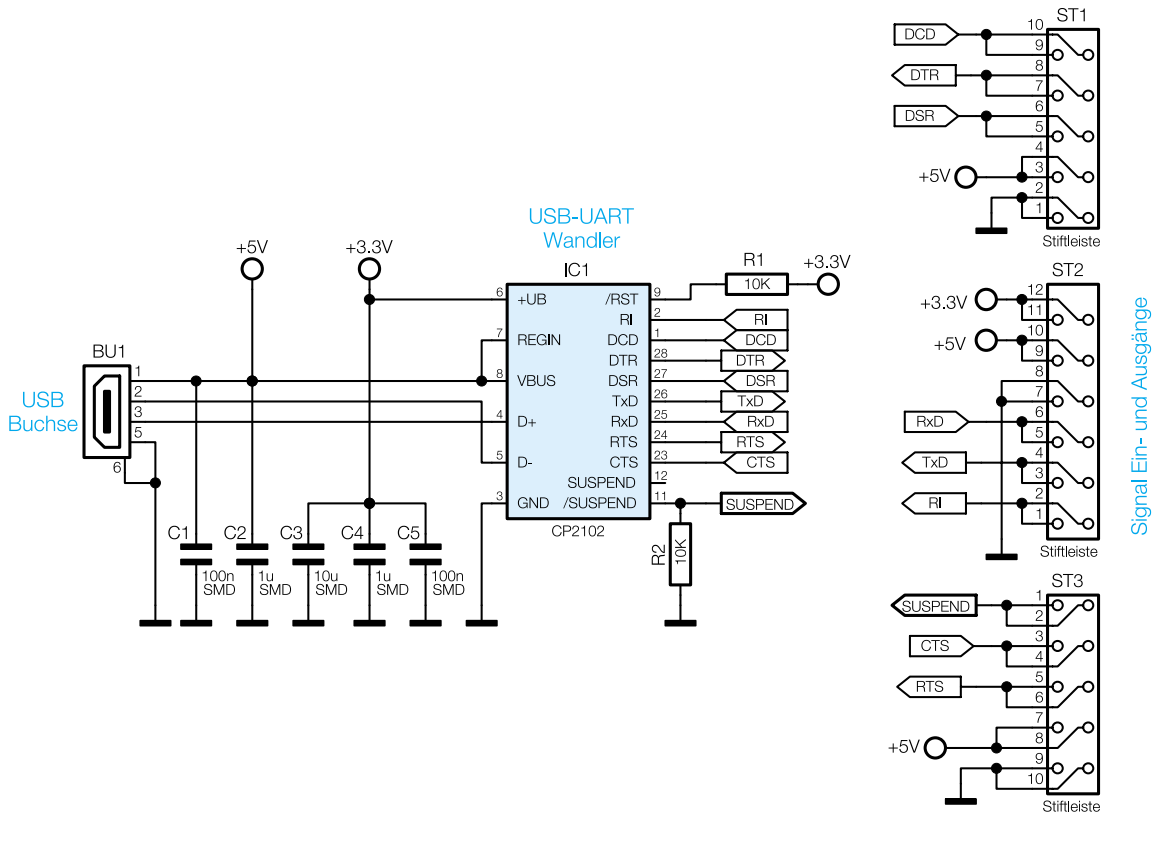
Bild 4: Die Schaltung des UM 2102
