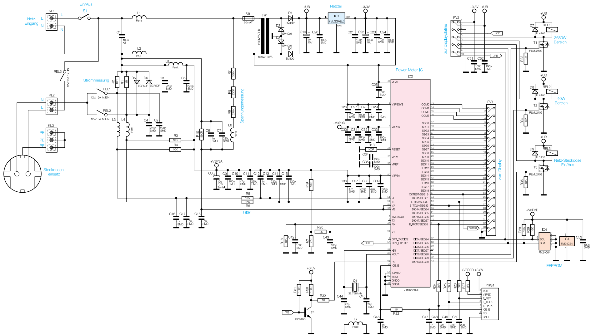
Bild 3: Hauptschaltbild des EA 8000
