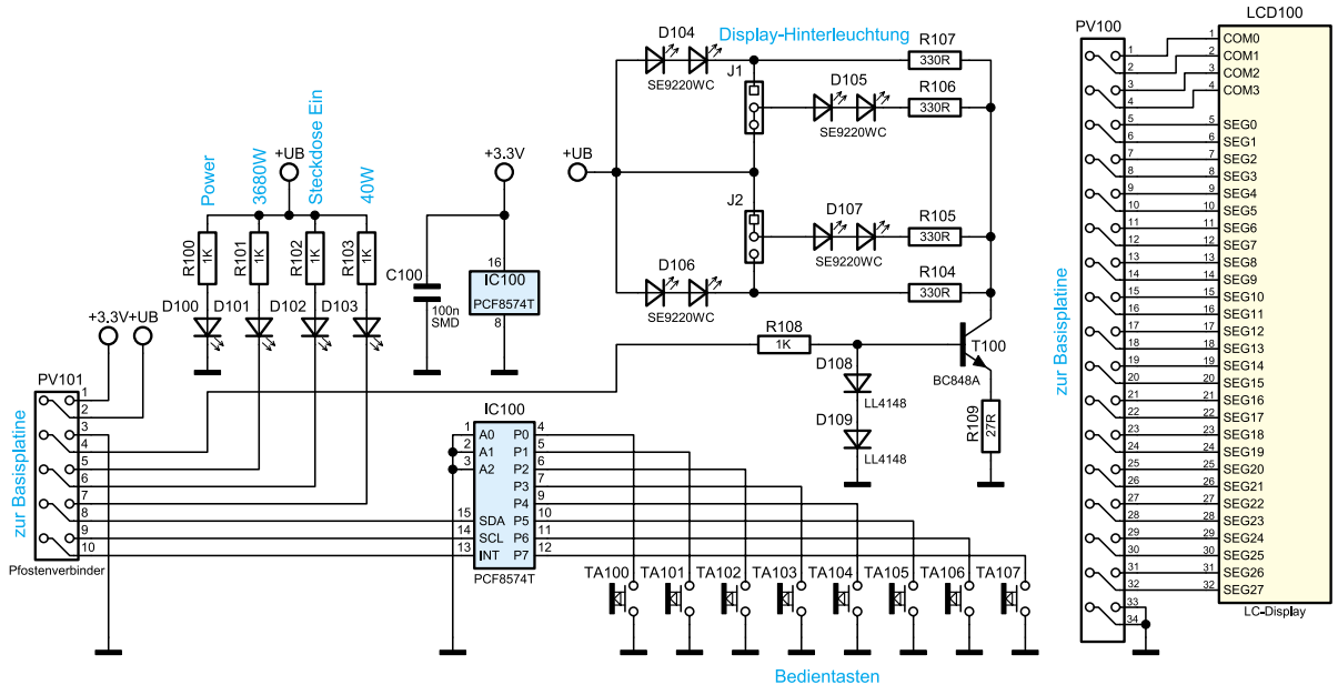
Bild 4: Bedien- und Anzeigeelemente des EA 8000
