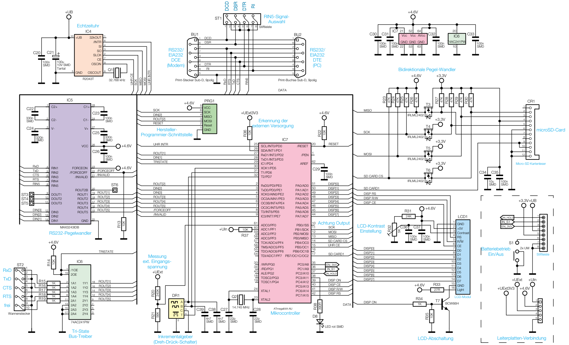
Bild 5: Das Hauptschaltbild des SDSSD1, das alle Bauelemente der Hauptplatine enthält.
