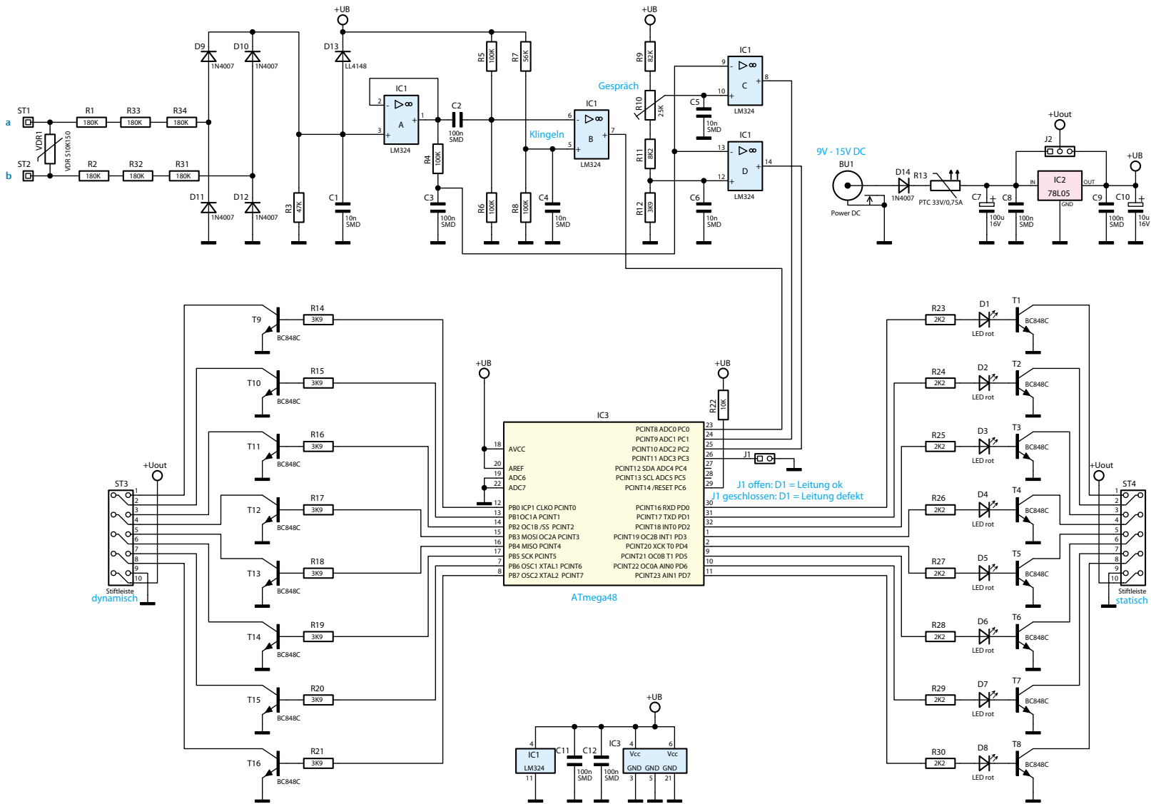
Bild 2: Die Schaltung des Telefon-Zustands-Melders
