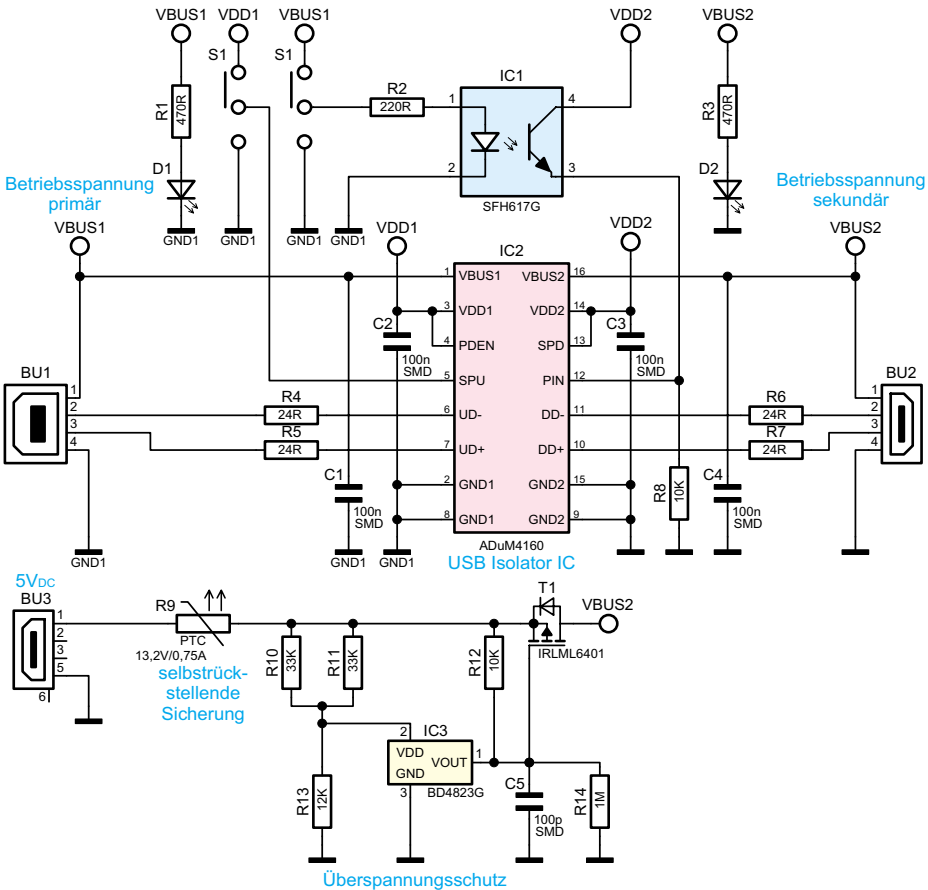
Bild 2: Die Schaltung des USB-Isolators UI 10
