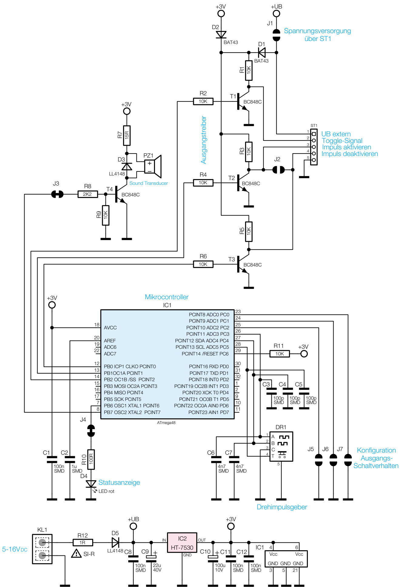
Bild 5: Schaltbild des ICS 100
