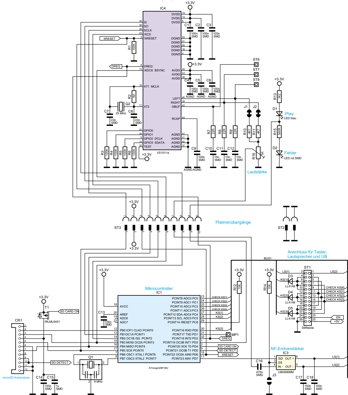
Bild 6: Hauptschaltbild
