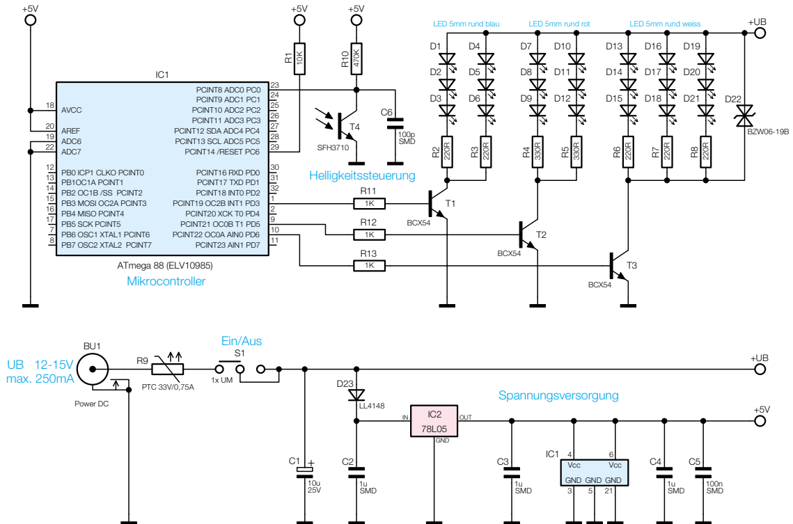
Bild 1: Schaltbild des TV-Simulators
