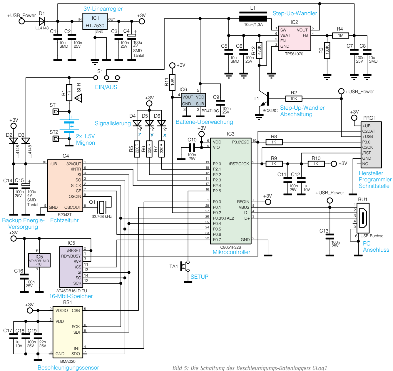
Bild 5: Die Schaltung des Beschleunigungs-Datenloggers GLog1
