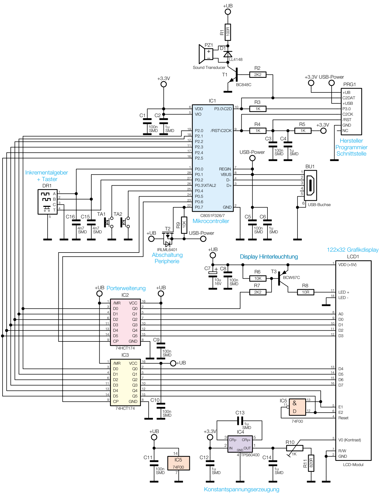
Bild 14: Die Schaltung des wakeoX-Terminals USB-BAT
