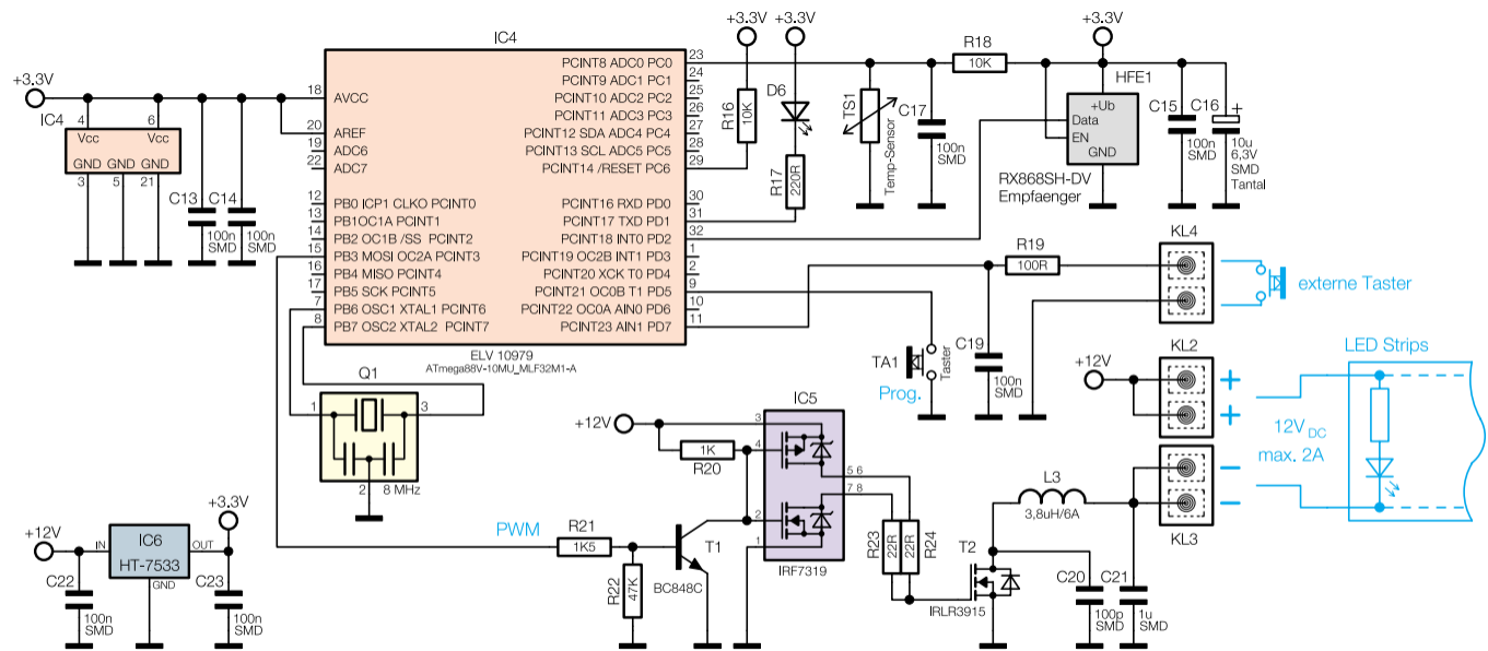
Bild 2: Das Schaltbild mit dem Steuerteil des FS20 LEDND
