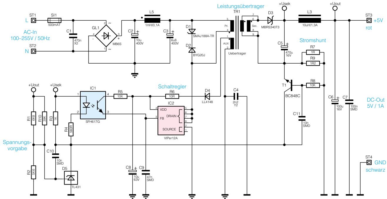
Bild 1: Schaltung des SPS05 M
