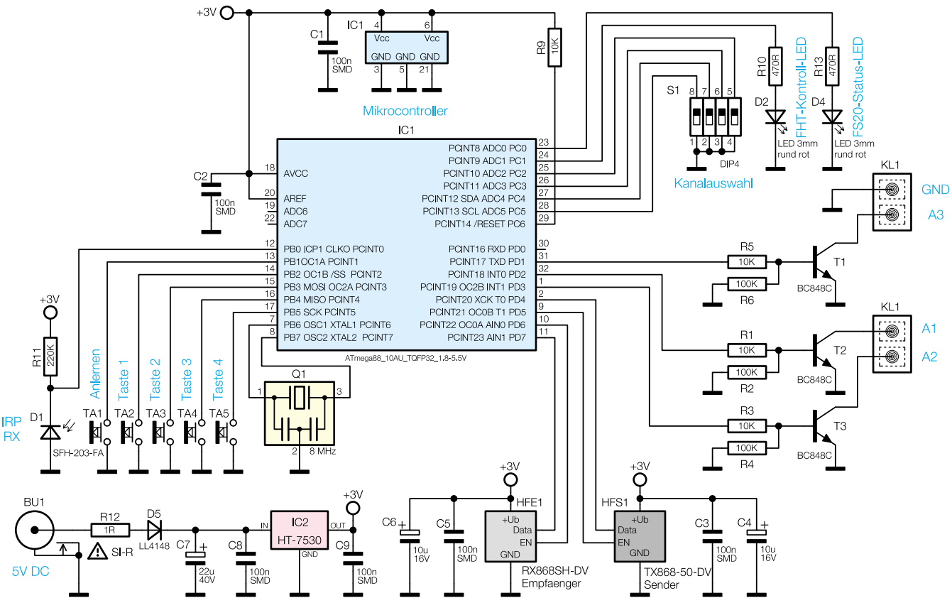
Bild 6: Schaltbild des FS20 TFI
