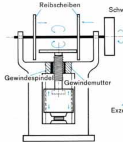
66.3 Reibspindelpresse
