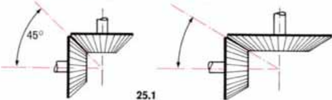
gleiche Zähnezahle
