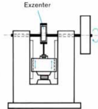
66.2 Doppelständer-Exzenterpresse
