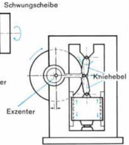
66.4 Kniehebelpresse
