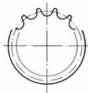
Zahnform für Kettenräder— Spezial-Kettenrad mit 15 Zähnen
