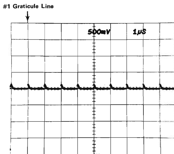
Fig. 7-5. 1 \mu s/DIV.
